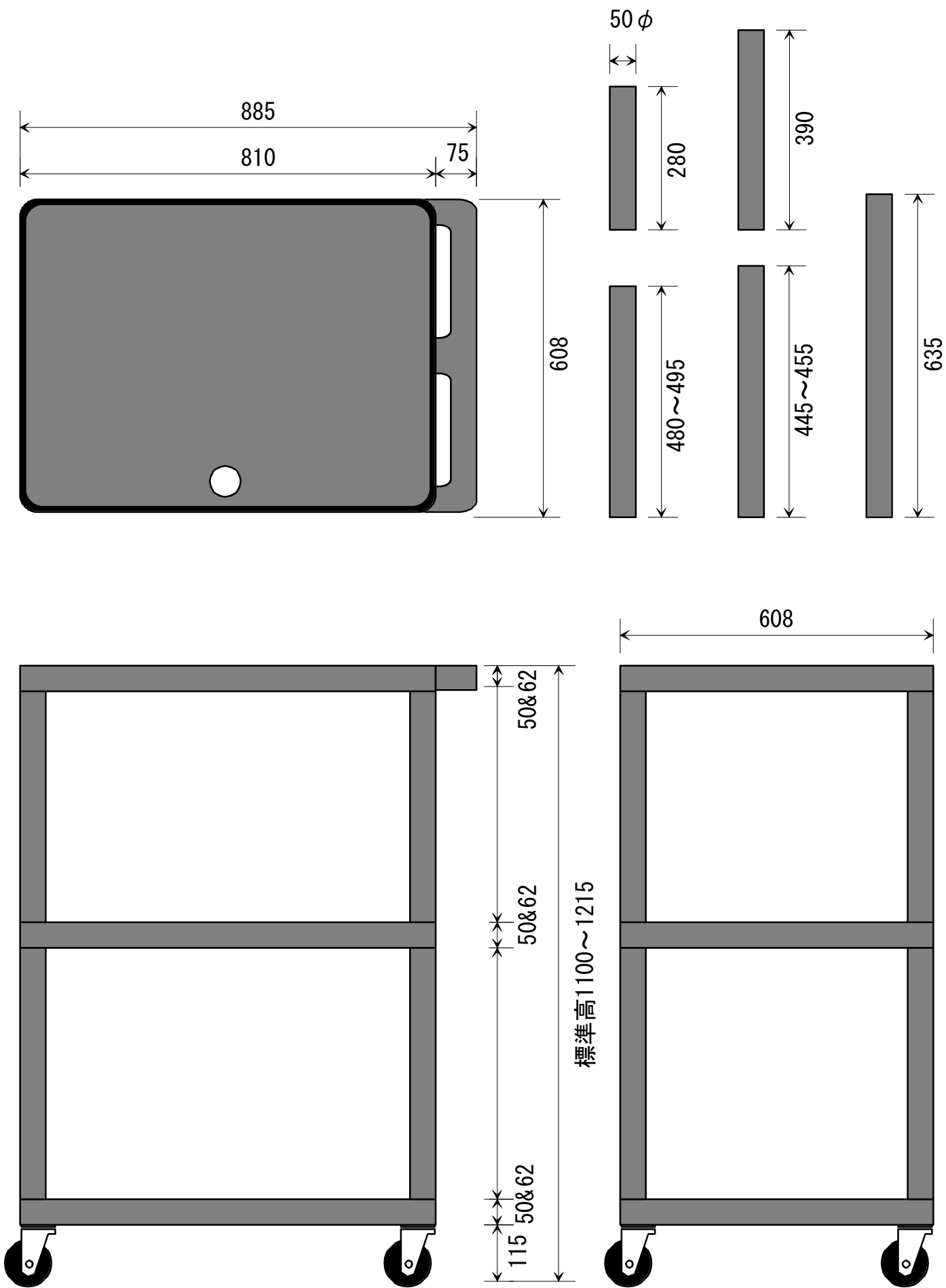
大型ラクサー台寸法図
