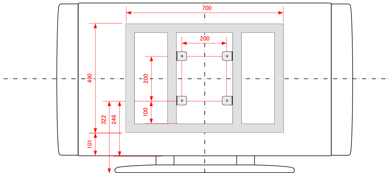
裏面金具穴位置
