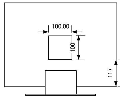
VESAマウント穴 (M4、深さ10mm)
